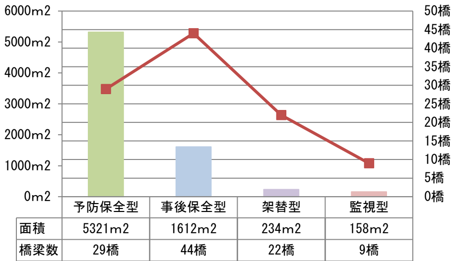
図 2-3-6 管理手法別橋面積比
